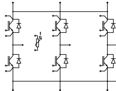
等效电路图
